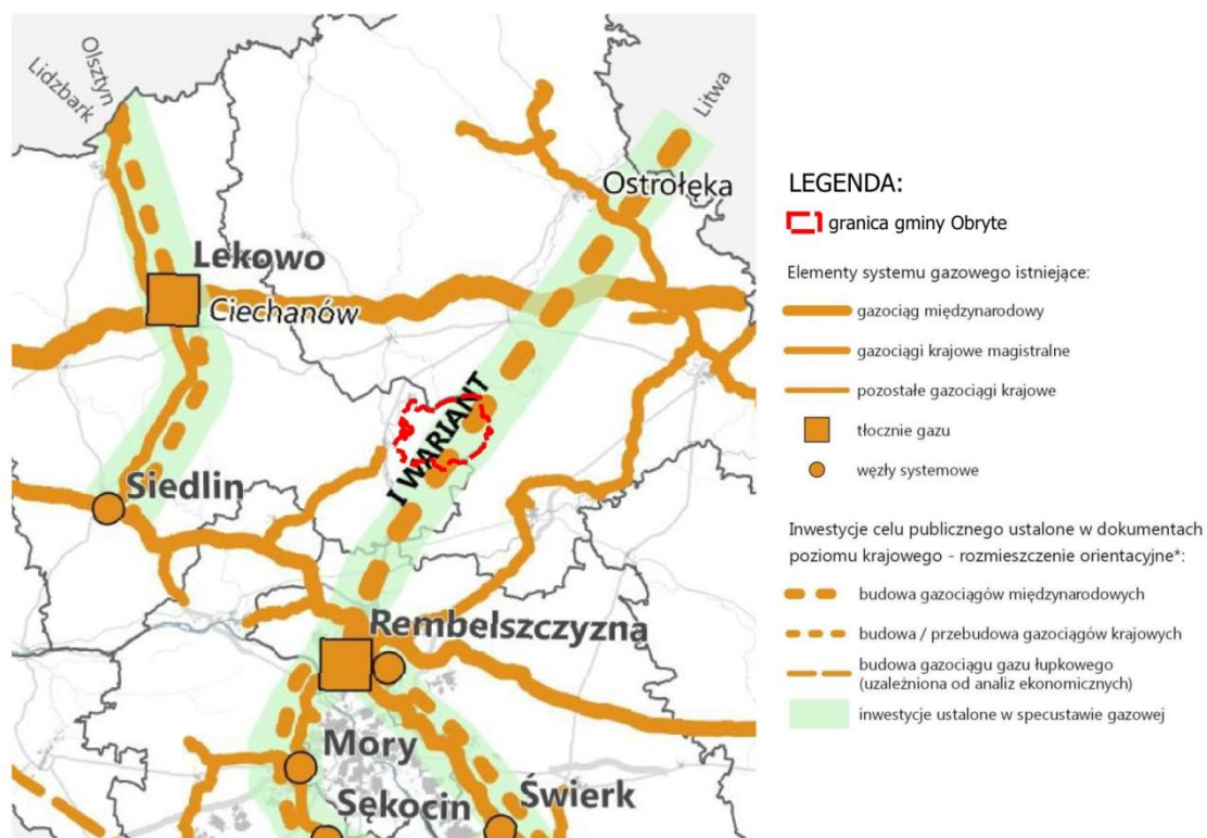
Rysunek 4. System gazowy wysokiego ciśnienia w rejonie gminy Obryte
